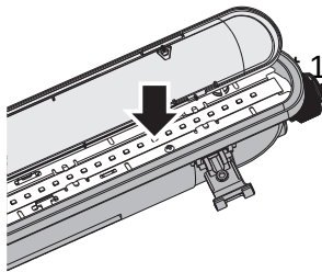
8. Close the luminaire
